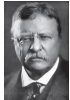
Теодор Рузвельт
